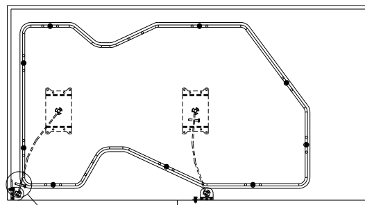
MONTAGEM DO PRODUTO INTERNO MÓVEL MÓDULO ABERTO
